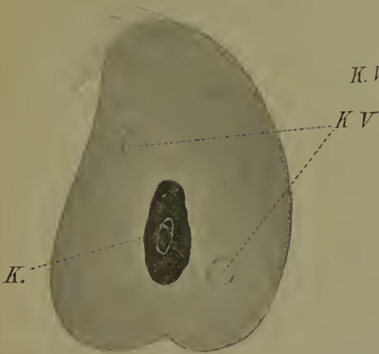
Fig. 86. Chilodon cyprini von der Rückenseite (nach Moroff).
